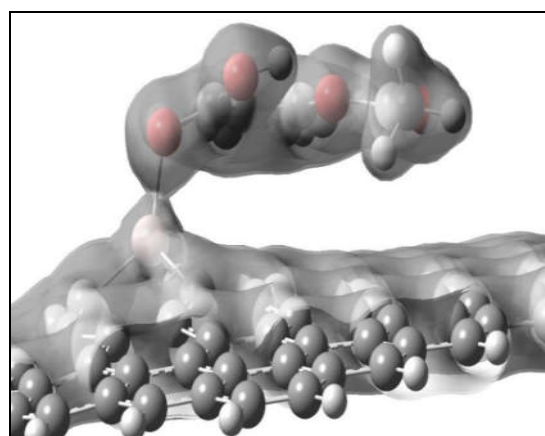
شکل ۹. تصویر توزیع دانسیته بار برای سیستم اسپیرین-گرافن آلاینده با آلومینیوم
