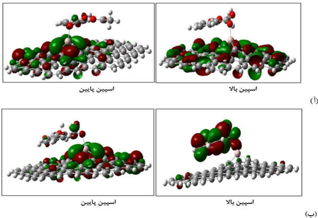
شکل ۸. تصویر اوربیتالهای مولکولی (آ) هومو و (ب) لومو در حالت‌های اسپین بالا و پایین برای سیستم اسپیرین-گرافن-آلومینیوم
