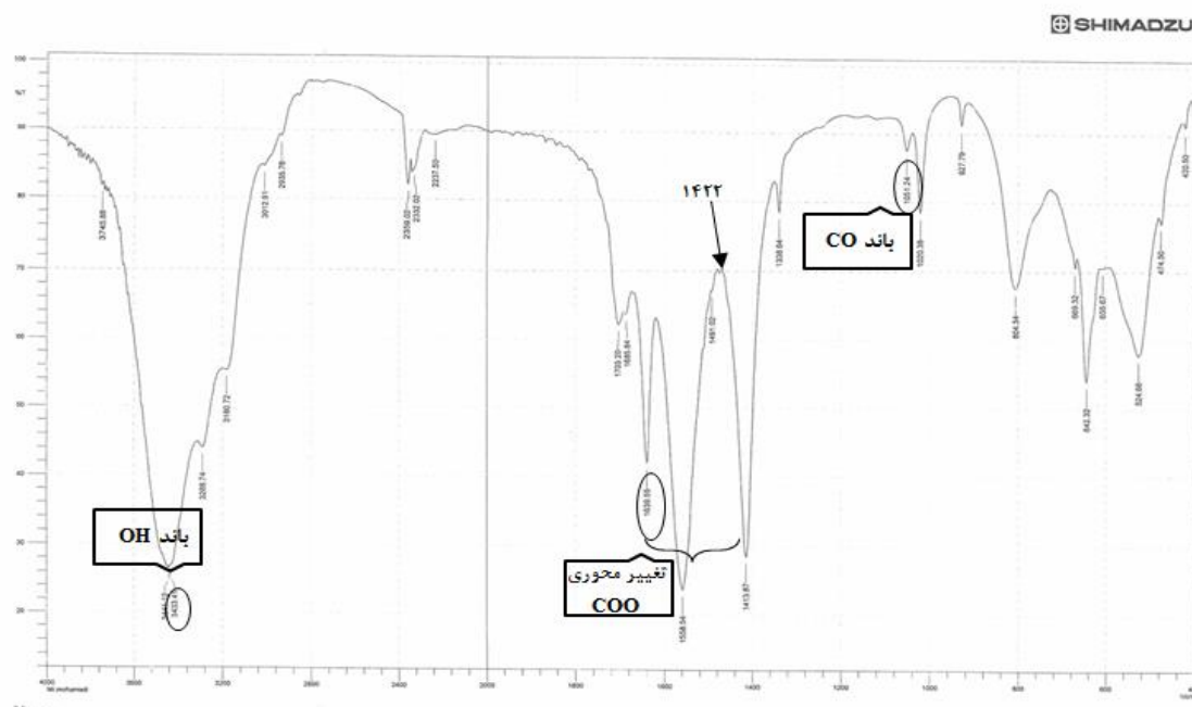
شکل ۳. اسپکتروفتوگرام مادون قرمز کربوکسی متیل کیتوزان و تری پلی فسفات با نسبت ۱:۱
