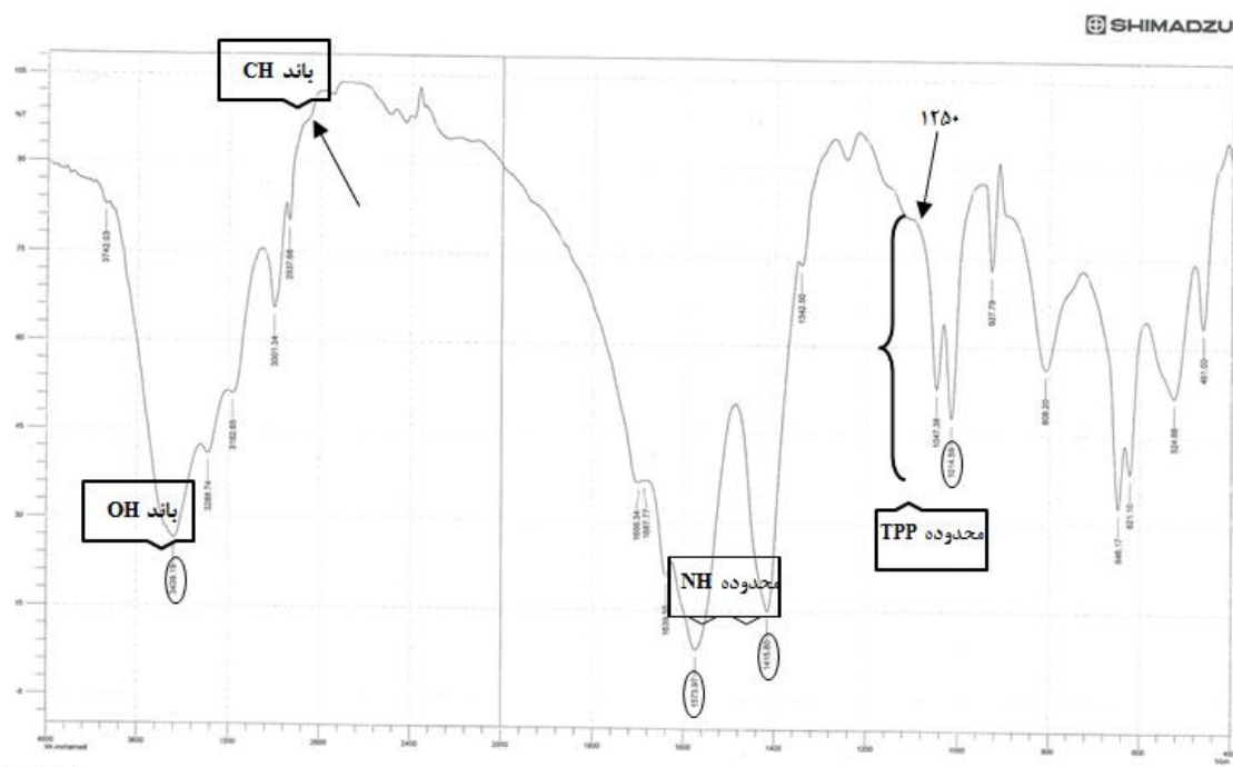
شکل ۲. اسپکتروفتوگرام مادون قرمز نانوذره کیتوزان/TPP با نسبت ۱:۱
