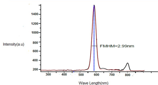
نمودار ۲. تحلیل یک خط طیفی خاص از عنصر هلیوم با طول موج حدود ۶۰۰ نانومتر. FWHM برابر ۲/۹۹ نانومتر بود.
