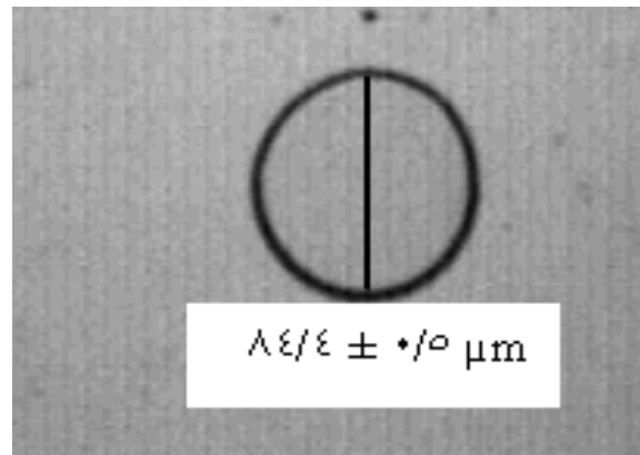
شکل 2- میانگین اندازه میکروکپسول‌ها در 300 rpm با بزرگنمایی 100×
