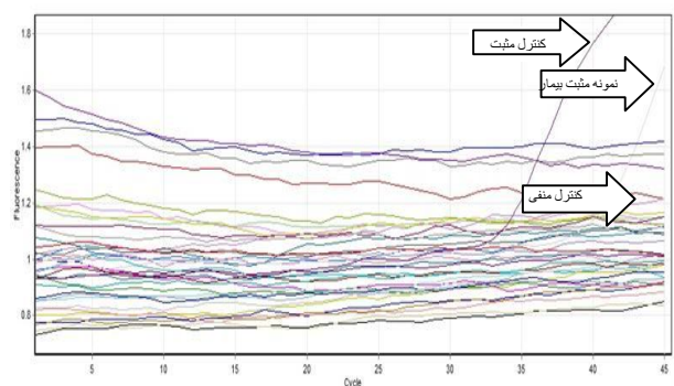
شکل ۳- منحنی‌های تکثیر نمونه‌های بیماران در آزمایش Real time PCR. همان طور که مشاهده می‌شود تنها کنترل مثبت و یکی از نمونه‌ها، میزان فلورسنت ساطع شده از آنها با افزایش مقادیر محصولات طی چرخه‌های واکنش PCR افزایش نشان می‌دهد.
