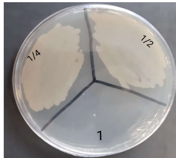
شکل ۳. نتایج اثردهی آنتی بیوتیک (مروپنم) بر روی باکتری پاتوژن. در رقت های ۱/۲ و ۱/۴ و کمتر رشد مشاهده و در رقت ۱ و بیشتر عدم رشد مشاهده شد.
