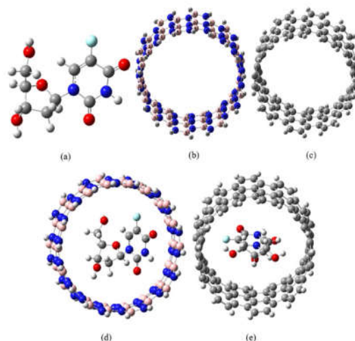
شکل ۱. ساختار بهینه (a) داروی فلوکسوریدین، (b) نانو لوله نیتريد بور (BNNT)، (c) نانولوله کربن (CNT)، (d) مخلوط دارو-نانولوله نیتريد بور (Floxuridine-BNNT)، (e) مخلوط دارو-نانولوله کربن (Floxuridine-CNT)
