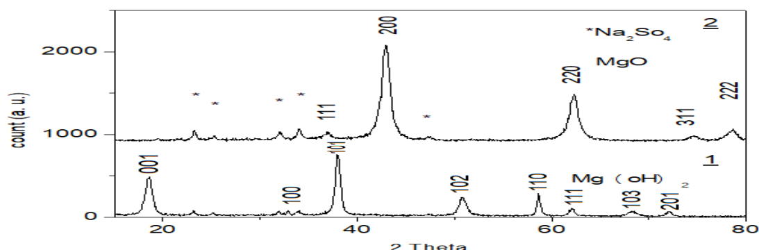
نمودار ۱. نمودار پراش پرتو X (XRD) به نانوذرات \text{MgO} جهت تعیین سایز
