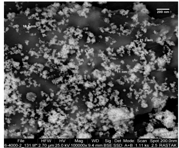
شکل ۱. طیف میکروسکوپ الکترونی SEM بدست آمده از نانوذره
