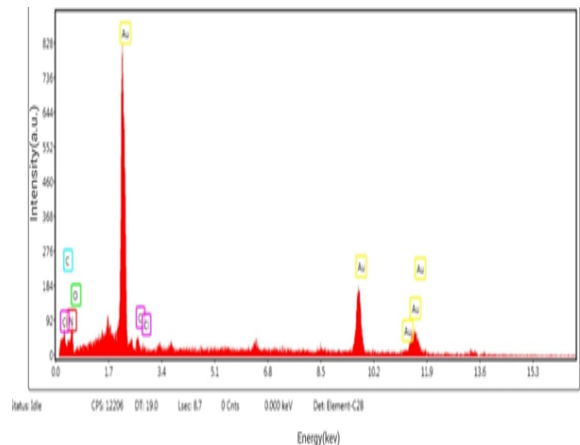
نمودار ۱. طیف EDX نانوذره. پیک های مربوط به Au، C، O و N وجود عناصر مذکور در نانوذره سنتز شده را تایید کرد.
