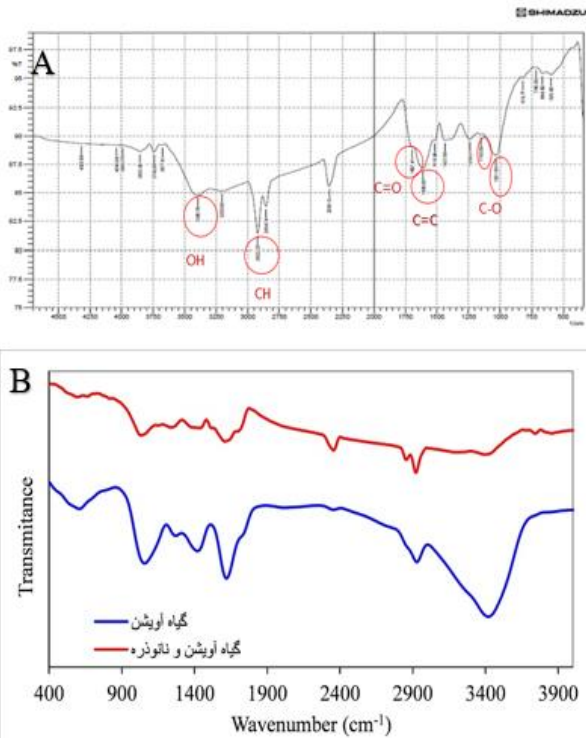
نمودار ۲. نمودار طیف مادون قرمز تبدیل فوریه (FTIR): A نمودار طیف مادون قرمز تبدیل فوریه نانوذره حاصل از تحقیق حاضر و B طیف مادون قرمز تبدیل فوریه گیاه آویشن به همراه نمودار تجمع
