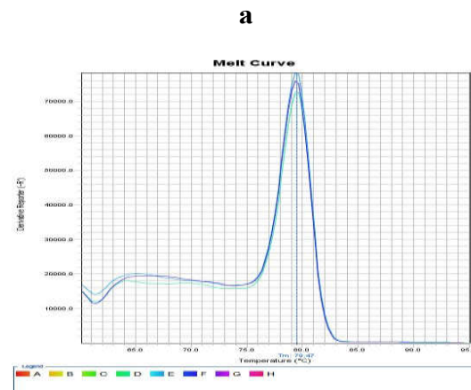
شکل ۴. منحنی ذوب قطعه تکثیرشده ژن Bad با نقطه ذوب (a) ۷۹/۴۷°C و ژن Gapdh دمای ذوب ۸۲/۴۶°C (b)
