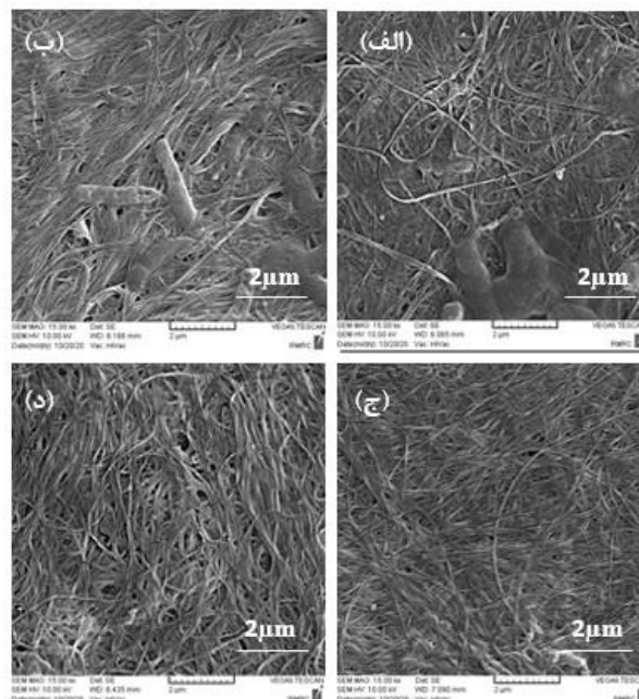
شکل ۳. تصویر میکروسکوپ الکترونی روبشی از نانوسلولز میکروبی خام و شبکه‌ای شده. الف) سلولز میکروبی خام، ب) سلولز میکروبی + اسید سیتریک ۰.۵٪ و سدیم هیپوفسفیت ۰.۲/۵٪، ج) سلولز میکروبی + اسید سیتریک ۰.۱٪ و سدیم هیپوفسفیت ۰.۵٪، د) سلولز میکروبی + اسید سیتریک ۰.۲٪ و سدیم هیپوفسفیت ۰.۱٪.
