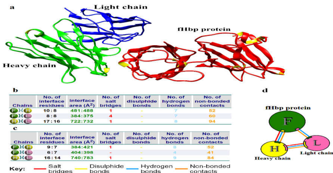
شکل ۱. داکینگ مولکولی دو فرم آنتی بادی هیبریدی با پروتئین fHbp، شکل (a) تصویر سه بعدی داکینگ مولکولی آنتی بادی هیبریدی با پروتئین fHbp، شکل (b) نتایج برهمکنش اسیده‌ای آمینه فرم هیبریدی (VL2-VH1) با آنتی ژن fHbp، شکل (c) نتایج برهمکنش اسیده‌ای آمینه فرم هیبریدی (VL2-VH1) با آنتی ژن fHbp، شکل (d) دیاگرام اتصال آنتی بادی هیبریدی فرم (VL2-VH1) با آنتی ژن
