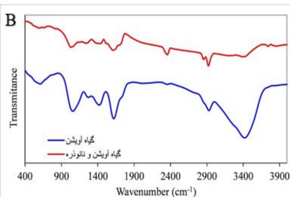
نمودار ۲. نمودار طیف مادون قرمز تبدیل فوریه (FTIR): نمودار A نمودار طیف مادون قرمز تبدیل فوریه نانوذره حاصل از تحقیق حاضر و B طیف مادون قرمز تبدیل فوریه گیاه آویشن به همراه نمودار تجمیع
