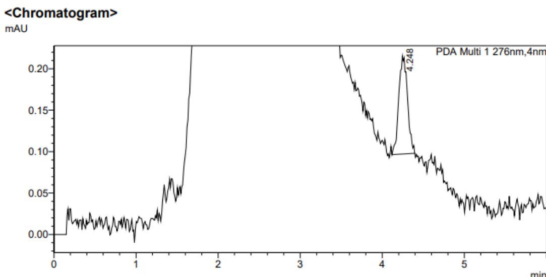
شکل ۴. کروماتوگرام مربوط به تزریق نمونه ۰/۰۲ میکروگرم در میلی لیتر آپیکسابان در پلاسما جهت تعیین حد تشخیص
